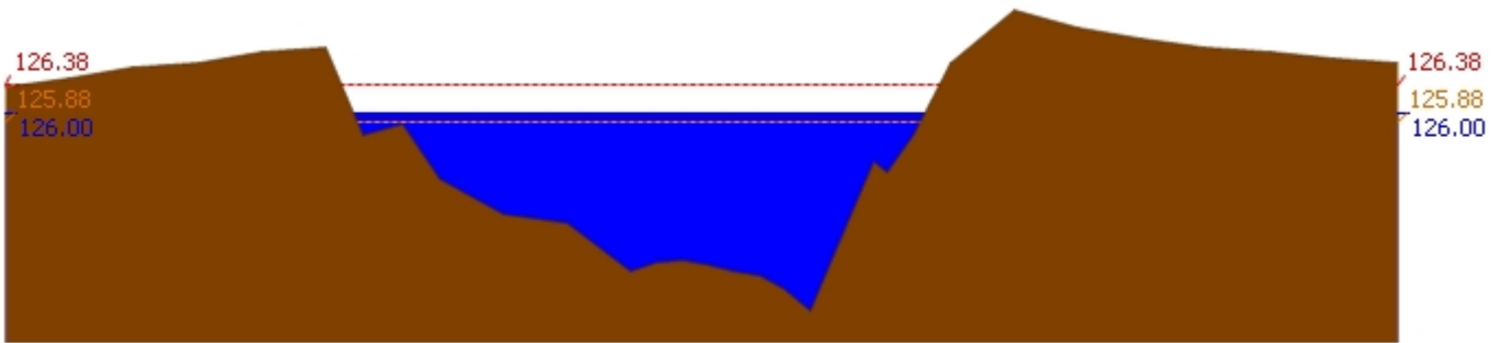
สถานี 110301T คลองโพธิ์ที่บ้านคลองบัวสามัคคี ต.ปางสวรรค์ อ.ชุมตาบง จ.นครสวรรค์ ระดับน้ำ 126.00 ม.รทก.
