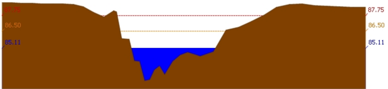
สถานี 110403T ฝายทับเสลาที่บ้านดินแดง ต.ประตู่หิน อ.ลานสัก จ.อุทัยธานี ระดับน้ำ 85.11 ม.รทก.
