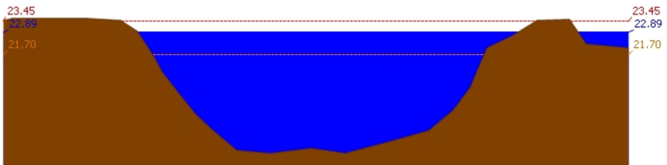
สถานี 110504T แม่น้ำตากแดดที่บ้านบุญลือ ต.เนินแจง อ.เมืองอุทัยธานี จ.อุทัยธานี ระดับน้ำ 22.89 ม.รทก.
