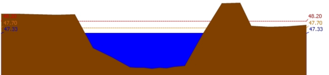
สถานี 110303T คลองโพธิ์ที่บ้านทุ่งสงบ ต.ไม้เขี้ยว อ.สว่างอารมณ์ จ.อุทัยธานี ระดับน้ำ 47.33 ม.รทก.
