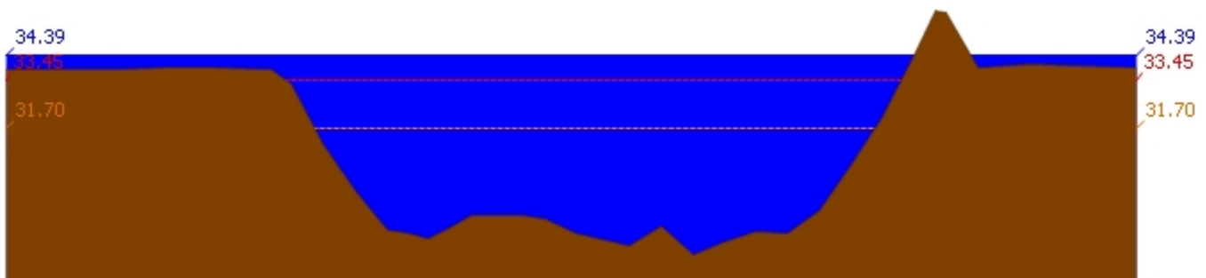
สถานี 110503T แม่น้ำตากแดดที่บ้านหนองขาลาย ต.หนองหลวง อ.สว่างอารมณ์ จ.อุทัยธานี ระดับน้ำ 34.39 ม.รทก.
