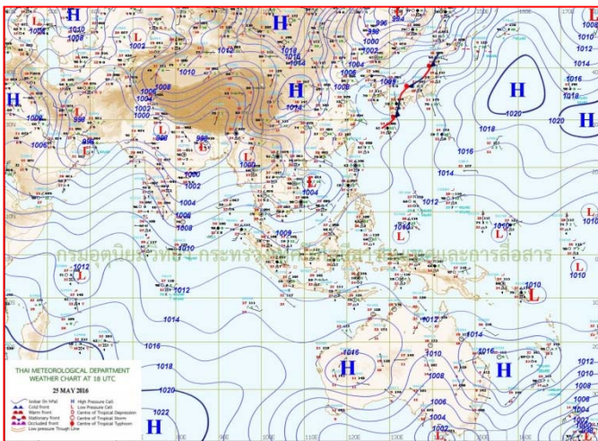
แผนที่อากาศ วันที่ ๒๖ พ.ค. ๒๕๕๙ เวลา ๐๖.๐๐ น.
