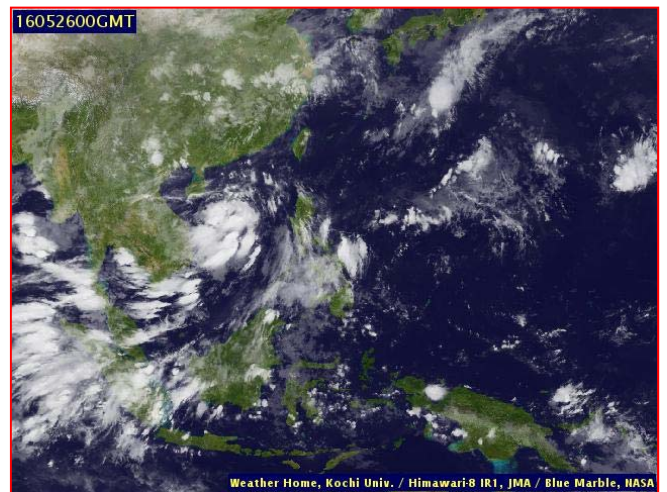
ภาพถ่ายจากดาวเทียม วันที่ ๒๖ พ.ค. ๒๕๕๙ เวลา ๐๗.๐๐ น.
