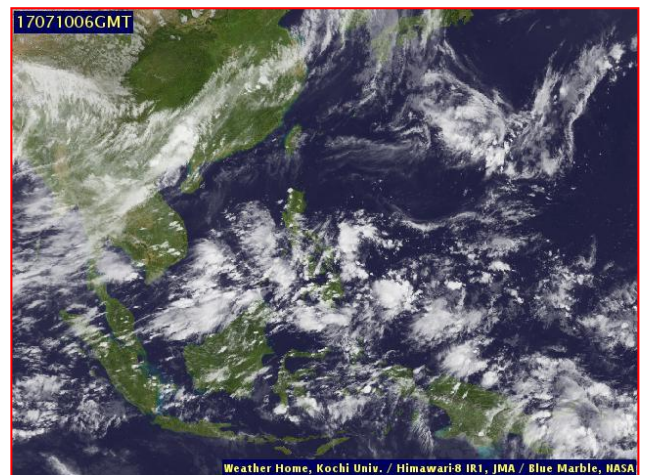
ภาพถ่ายจากดาวเทียม วันที่ ๑๐ ก.ค. ๒๕๖๐ เวลา ๑๓.๐๐ น.
