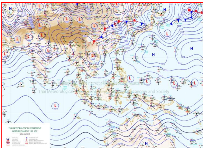
แผนที่อากาศ วันที่ ๑๐ ก.ค. ๒๕๖๐ เวลา ๐๗.๐๐ น.
