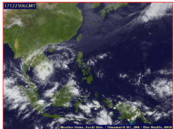
ภาพถ่ายจากดาวเทียม วันที่ ๒๕ ธ.ค. ๒๕๖๐ เวลา ๑๓.๐๐ น.
