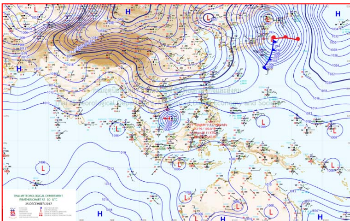
แผนที่อากาศ วันที่ ๒๕ ธ.ค. ๒๕๖๐ เวลา ๐๗.๐๐ น.
