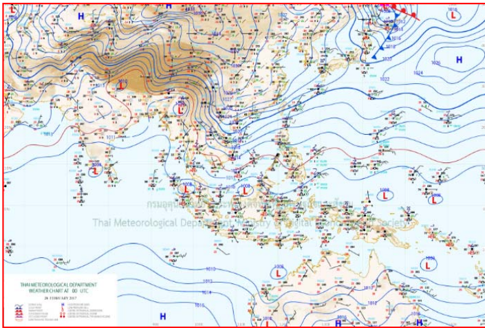
แผนที่อากาศ วันที่ ๒๖ ก.พ. ๒๕๖๐ เวลา ๐๗.๐๐ น.
