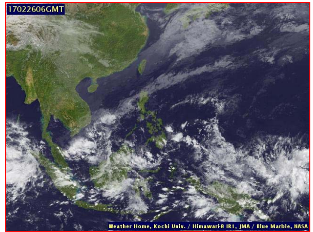
ภาพถ่ายจากดาวเทียม วันที่ ๒๖ ก.พ. ๒๕๖๐ เวลา ๑๓.๐๐ น.
