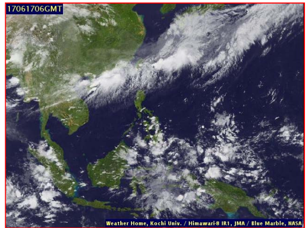
ภาพถ่ายจากดาวเทียม วันที่ ๑๗ มิ.ย. ๒๕๖๐ เวลา ๑๓.๐๐ น.
