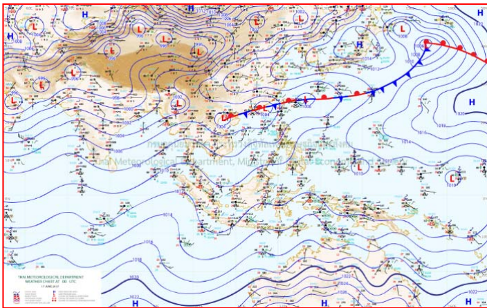
แผนที่อากาศ วันที่ ๑๗ มิ.ย. ๒๕๖๐ เวลา ๑๒.๐๐ น.
