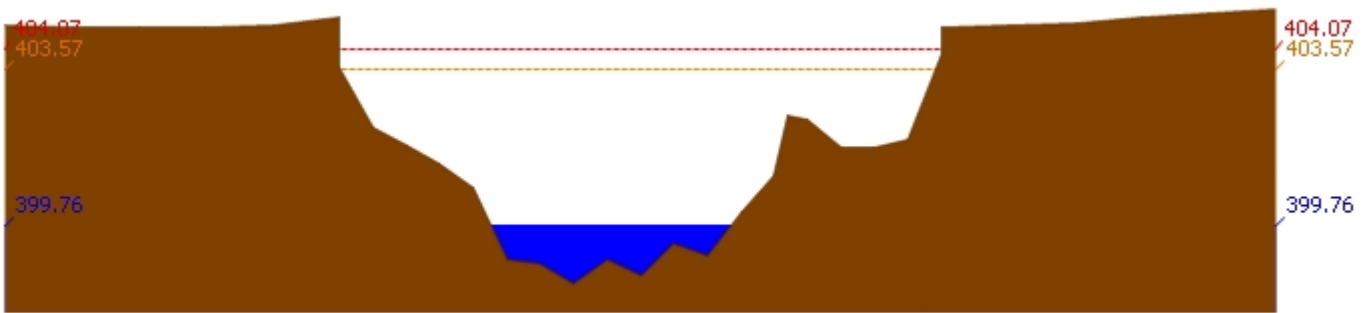
สถานี 070110T แม่น้ำวังที่ อ.วังเหนือ ต.วังเหนือ อ.วังเหนือ จ.ลำปาง ระดับน้ำ 399.76 ม.รทก.
