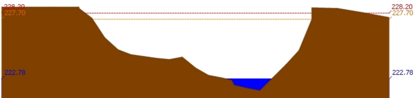
สถานี 070703T น้ำแม่ตำที่บ้านนาบอน ต.ทุ่งงาม อ.เสริมงาม จ.ลำปาง ระดับน้ำ 222.78 ม.รทก.
