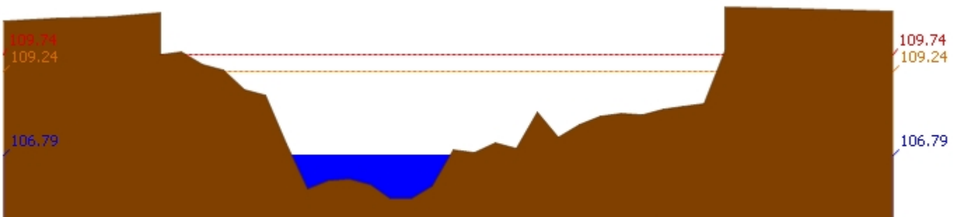
สถานี 061701T ห้วยแม่ท้อที่อำเภอเมืองตาก ต.แม่ท้อ อ.เมืองตาก จ.ตาก ระดับน้ำ 106.79 ม.รทก.
