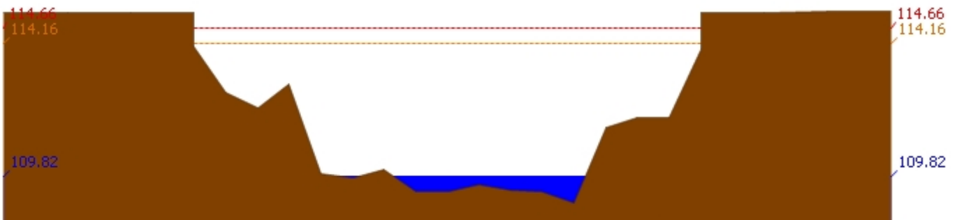
สถานี 061801T คลองวังเจ้าที่บ้านคลองลึก ต.เชียงทอง อ.วังเจ้า จ.ตาก ระดับน้ำ 109.82 ม.รทก.
