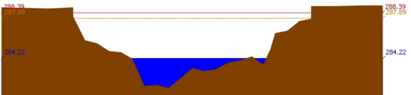
สถานี 070111T แม่น้ำวังที่บ้านโป่งชัย ต.บ้านเสา อ.แจ้ห่ม จ.ลำปาง ระดับน้ำ 284.22 ม.รทก.
