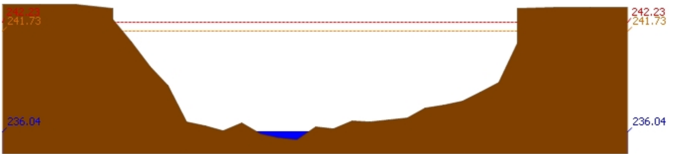
สถานี 070114T แม่น้ำวังที่บ้านปางชัย ต.บ้านเสด็จ อ.เมืองลำปาง จ.ลำปาง ระดับน้ำ 236.04 ม.รทก.
