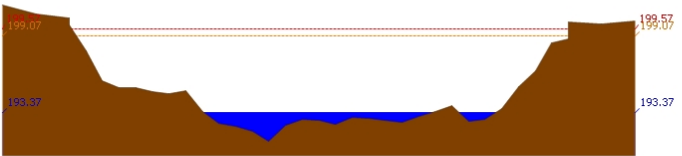
สถานี 070115T น้ำแม่วังที่บ้านอ้อ ต.แม่แก้ว อ.สบปราบ จ.ลำปาง ระดับน้ำ 193.37 ม.รทก.
