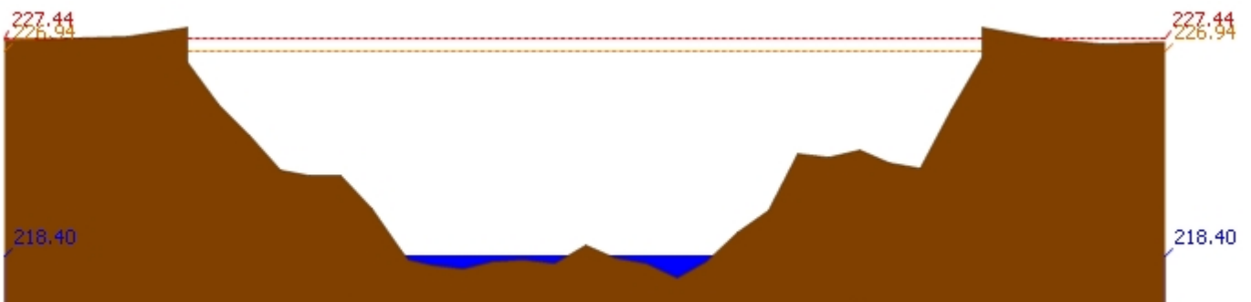
สถานี 070113T แม่น้ำวังที่ จ.ลำปาง ต.เวียงเหนือ อ.เมืองลำปาง จ.ลำปาง ระดับน้ำ 218.40 ม.รทก.
