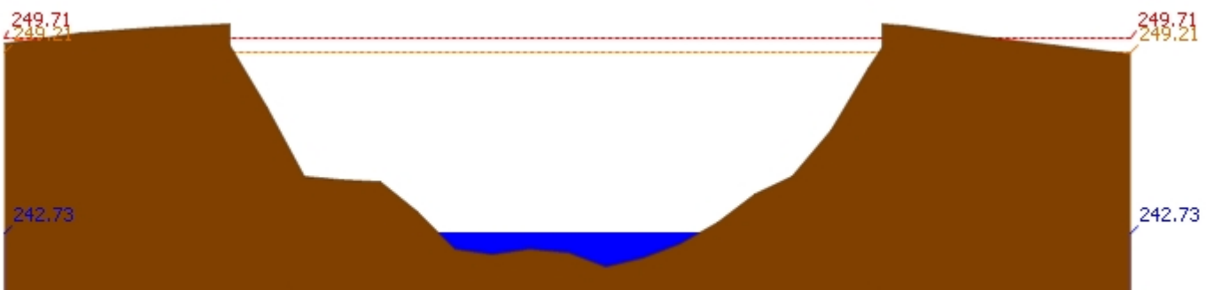
สถานี 070112T แม่น้ำวังที่บ้านบุญนา ต.บุญนาพัฒนา อ.เมืองลำปาง จ.ลำปาง ระดับน้ำ 242.73 ม.รทก.
