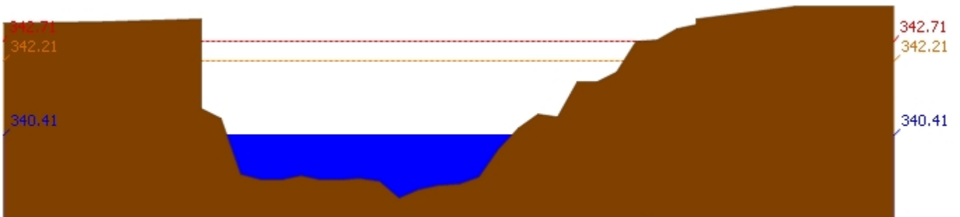
สถานี 070304T น้ำแม่สอยที่บ้านหนองกอก ต.แม่สอก อ.แจ้ห่ม จ.ลำปาง ระดับน้ำ 340.41 ม.รทก.
