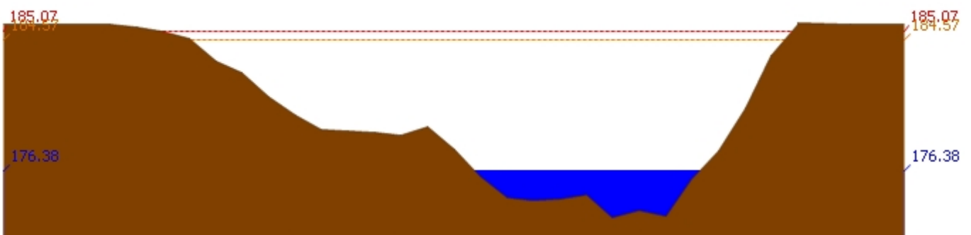
สถานี 070116T แม่น้ำวังที่บ้านแม่เตี๊ยะ ต.แม่ถอด อ.เถิน จ.ลำปาง ระดับน้ำ 176.38 ม.รทก.
