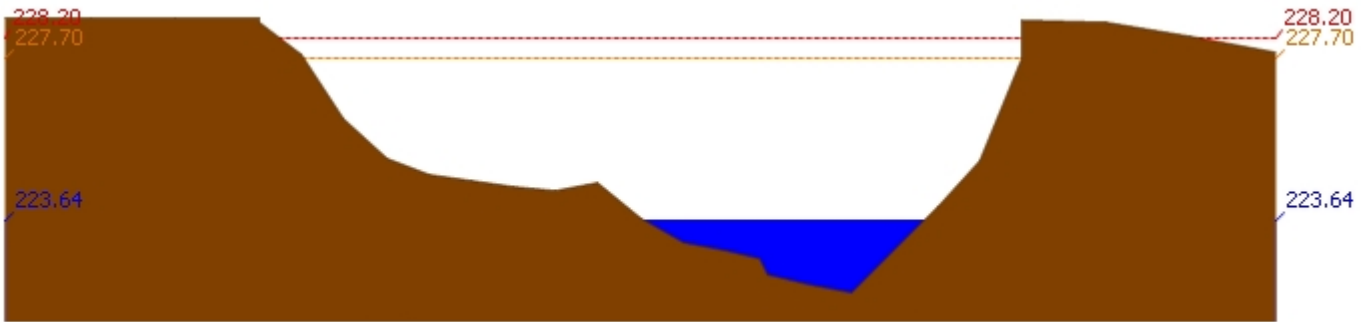
สถานี 070703T น้ำแม่ต้าที่บ้านนาบอน ต.ทุ่งงาม อ.เสริมงาม จ.ลำปาง ระดับน้ำ 223.64 ม.รทก.
