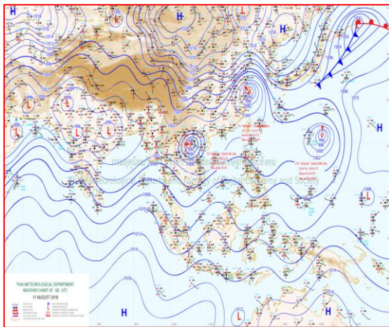
แผนที่อากาศ วันที่ 17 ส.ค. 2561 เวลา 07.00 น.
