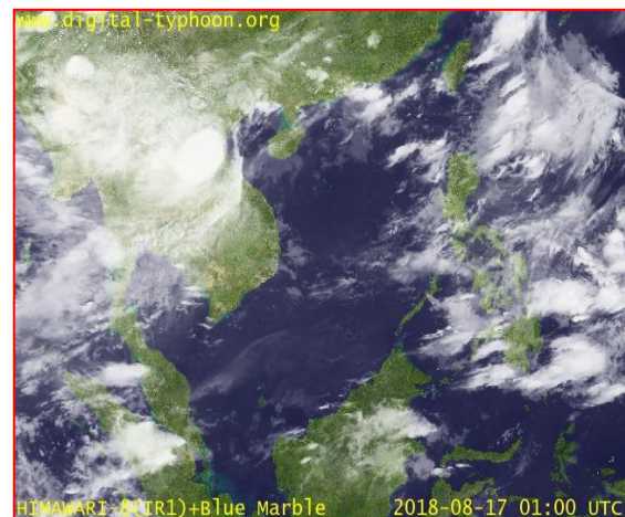
ภาพถ่ายจากดาวเทียม วันที่ 17 ส.ค. 2561
