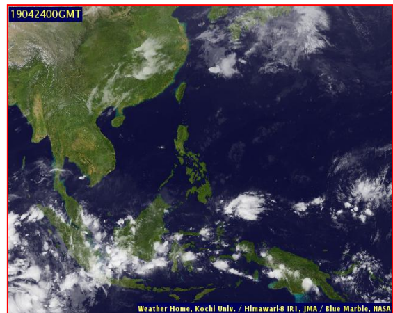
ภาพถ่ายจากดาวเทียม วันที่ 24 เม.ย. 2562
