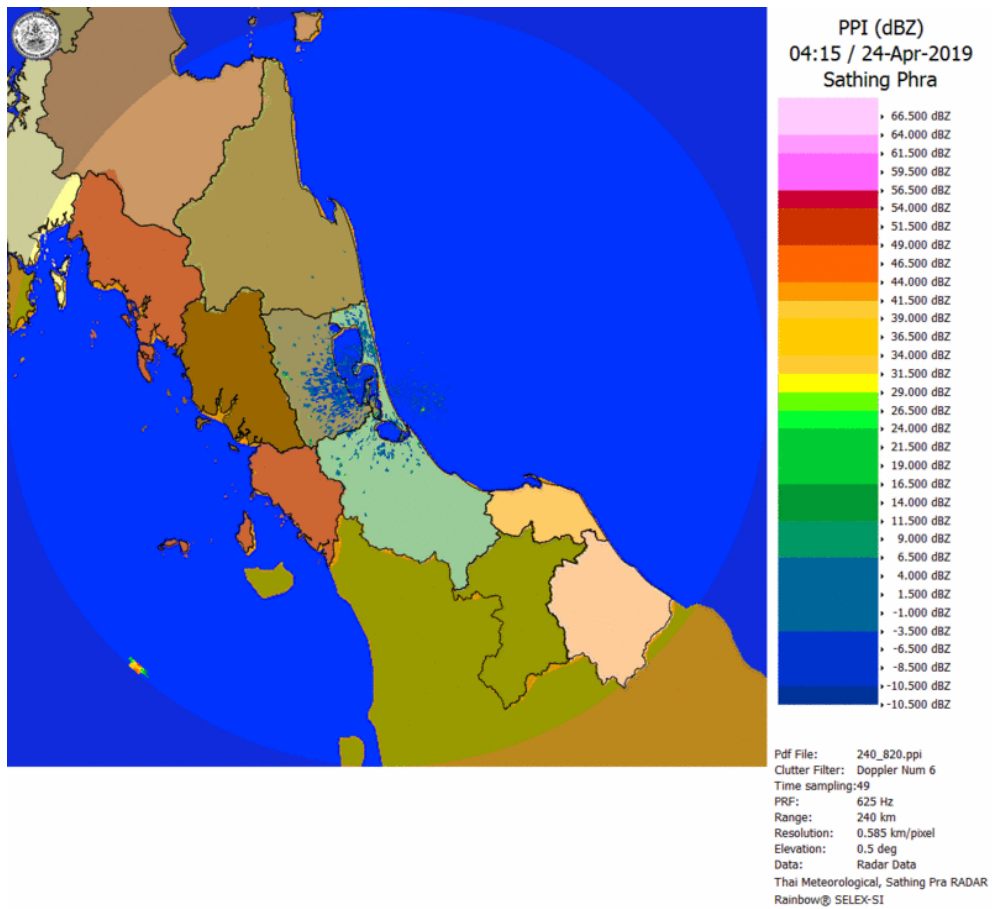
ภาพเรดาร์ตรวจอากาศ “สทิงพระ” ณ วันที่ 24 เมษายน 2562 (ที่มา : กรมอุตุนิยมวิทยา)
