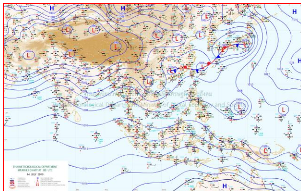
แผนที่อากาศ วันที่ 14 ก.ค. 2562 เวลา 07.00 น.
