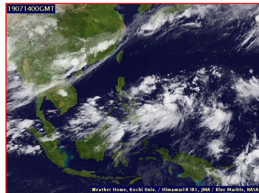
ภาพถ่ายจากดาวเทียม วันที่ 14 ก.ค. 2562
